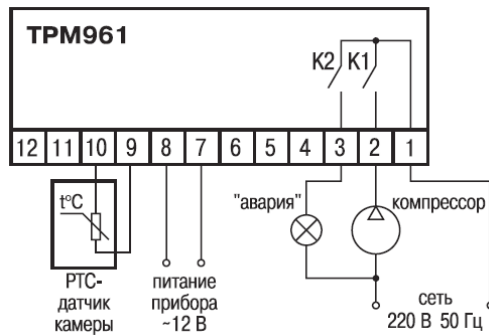
Рис. Б.1 – Схема подключения прибора
