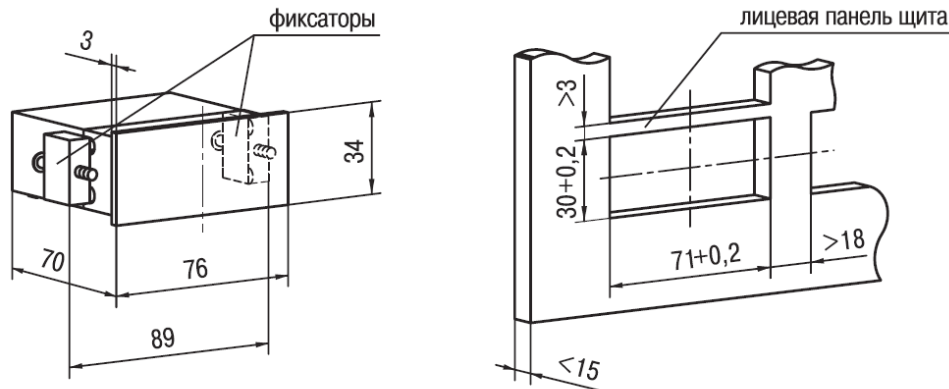
Рисунок А.1 – Габаритные и установочные размеры прибора
