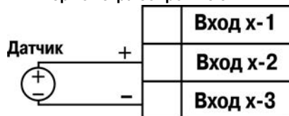
Рисунок Б.4 - Схема подключения активного датчика с выходом в виде напряжения -50.0...50.0 мВ или 0...1.0 В
