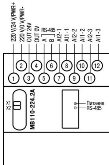
Рисунок Б.1 - Общий чертеж MB110-2A
