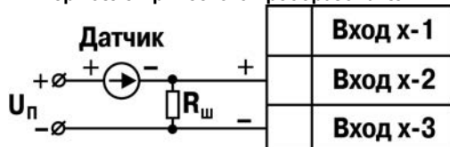
Рисунок Б.5 - Схема подключения активного датчика с токовым выходом 0...5, 0...20 или 4...20 мА ( R_{ш}=50,000 \pm 0,025 \text{ Ом} )
